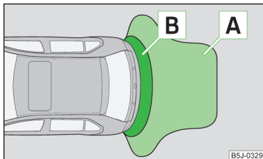
Fig. 113 Asistența la parcare: Raza de acțiune a senzorilor
