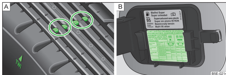
Fig. 133 Prezentarea în principiu: Profilul anvelopei cu indicatoare de uzură / clapeta rezervorului deschisă cu un tabel al dimensiunilor și presiunilor din anvelope
