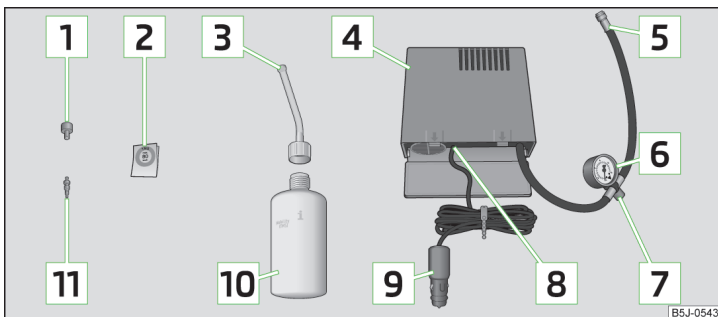
Fig. 145 Prezentarea în principiu: Componentele setului de depanare
