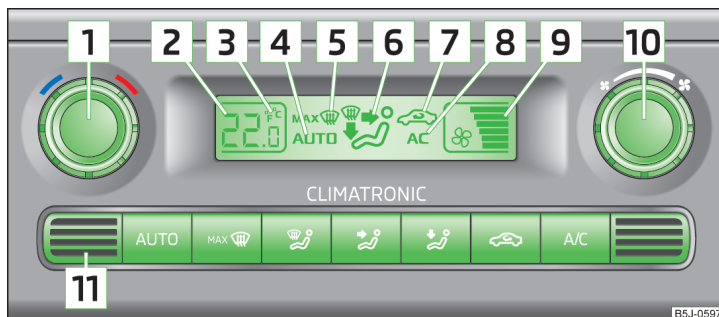
Fig. 97 Climatronic: Elementele de comandă
