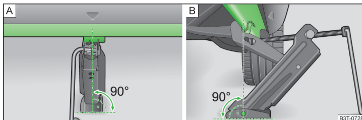
Fig. 143 aplicarea cricului
