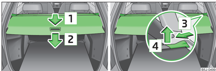
Fig. 66 Portbagajul: Masca rulată a portbagajului / Demontarea măștii rulante a portbagajului
