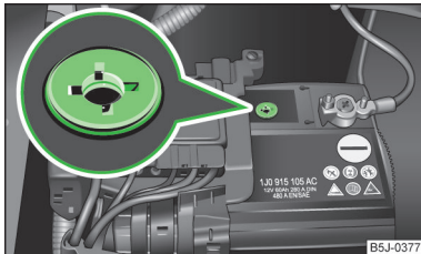
Fig. 132 Bateria autovehiculului: Indicatorul nivelului electrolitului
