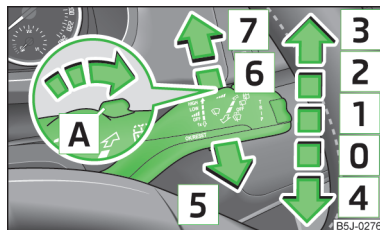
Fig. 50 Maneta: Pozițiile ștergătoarelor de parbriz și instalației de spălare a parbrizului
