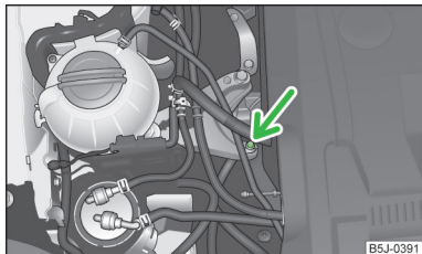
Fig. 147 Punctul de masă al motorului: Sistemul START-STOP
