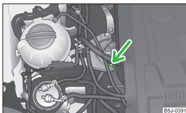
Fig. 147 Compartimentul motor: Punctul de masă
