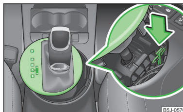
Fig. 91 Deblocarea de urgență a selectorului de viteze
