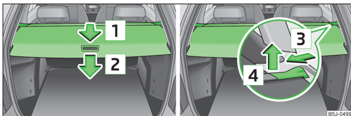
Fig. 49 Portbagajul: Masca rulantă a portbagajului / Demontarea măștii rulante a portbagajului
