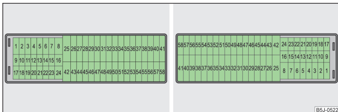
Fig. 151 Reprezentare schematică a panoului de siguranțe pentru autovehi- culele cu volanul pe stânga / dreapta
