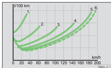
Fig. 92 Prezentarea în principiu: Consumul de combustibil în l/100 km în funcție de treapta de viteză cuplată
