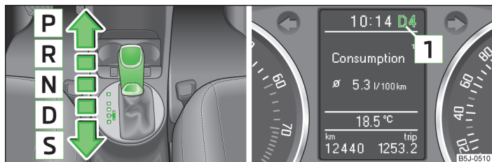
Fig. 89 Selectorul de viteze / Afișaj MAXI DOT Pozițiile selectorului de viteze
