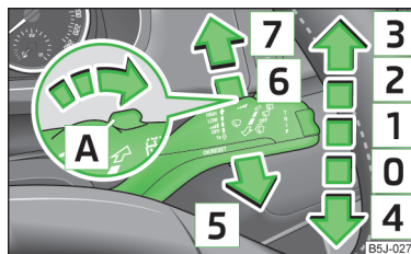
Fig. 33 Maneta: Pozițiile ștergătoarelor de parbriz și instalației de spălare a parbrizului
