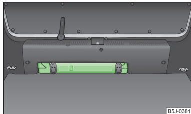
Fig. 138 Amplasarea triunghiului reflectorizant
