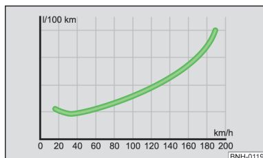
Fig. 93 Prezentarea în principiu: Consumul de combustibil în l/100 km și viteza în km/h
