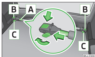
Fig. 56 Montarea suportului transversal
