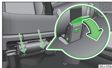
Fig. 139 Extinctorul
