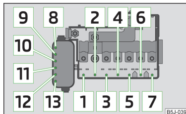
Fig. 152 Bateria autovehiculului: Capacul panoului de siguranțe
