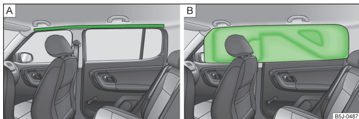
Fig. 115 Locul de amplasare a airbagului cortină / airbag cortină umplut cu gaz
