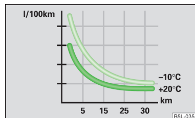
Fig. 94 Prezentarea în principiu: Consumul de combustibil în l/100 km la diverse temperaturi
