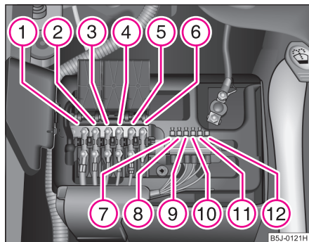
Fig. 170 Reprezentare schematică a dispoziției siguranțelor de pe baterie
