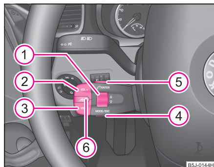
Fig. 99 Modul multifuncțional: Taste pentru radio și telefon
