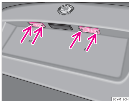
Fig. 177 Demontarea lămpii numărului de înmatriculare
