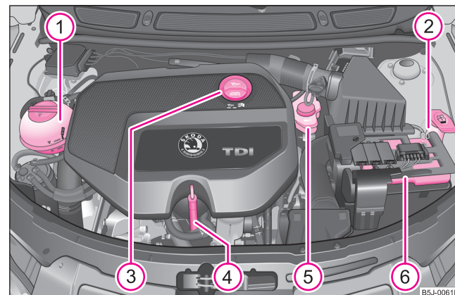
Fig. 144 Motorul diesel 1,9 l/77 kW
