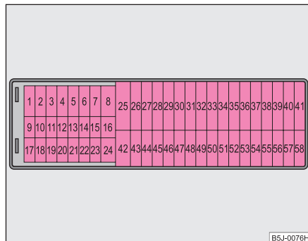
Fig. 167 Prezentare schematică a suportului de siguranțe
