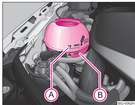
Fig. 146 Compartimentul motor: Vasul de expansiune al lichidului de răcire
