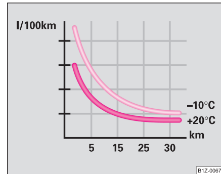
Fig. 138 Consumul de carburant în l/100 km la diverse temperaturi
