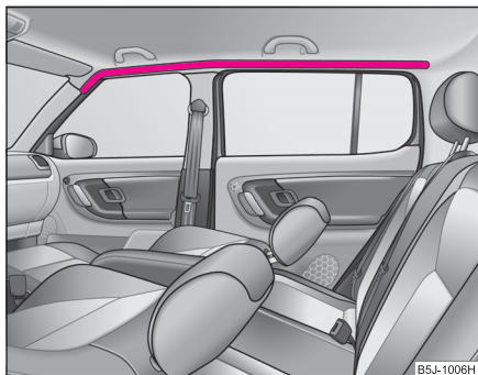
Fig. 119 Amplasarea airbag-urilor cortină
