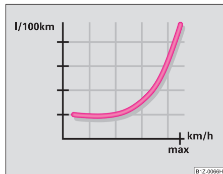
Fig. 137 Consumul de carburant în l/100 km și viteza în km/h
