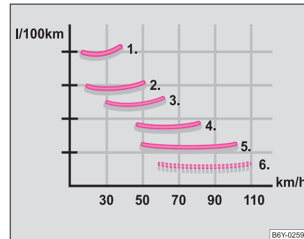
Fig. 136 Consumul de carburant în l/100 km și viteza în km/h
