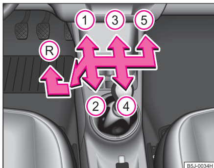
Fig. 90 Schemă de comutare la autovehiculele cu transmisie manuală cu 5 viteze
