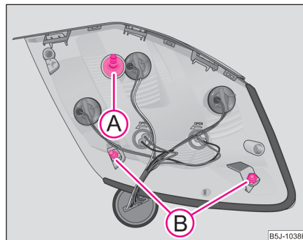
Fig. 179 Montarea lămpii din spate
