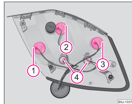
Fig. 180 Lampa din spate: Poziția becurilor
