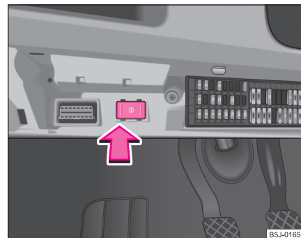
Fig. 35 Compartimentul siguranțelor: înterupătorul pentru lumina de zi
