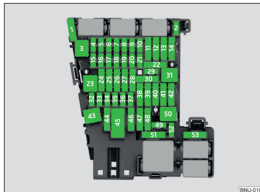
Fig. 334 Siguranțe
