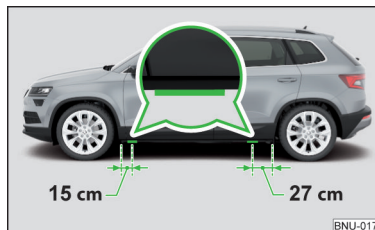
Fig. 314 Nervuri de fixare pentru cric
