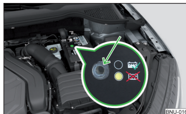
Fig. 302 Bateria autovehiculului: Indicatorul nivelului electrolitului
