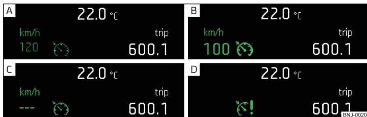
Fig. 268 Afişajul panoului de bord: Exemple de afişări de stare a sistemului de menținere automată a vitezei de deplasare (GRA)
