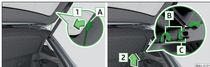
Fig. 135 Scoaterea măștii portbagajului
