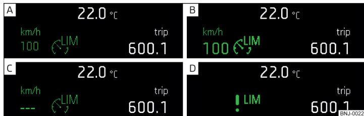
Fig. 270 Afișajul panoului de bord: Exemple de afișări de stare ale limitatorului de viteză
