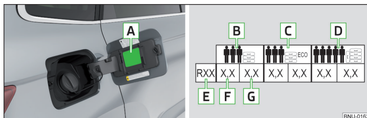
Fig. 303 Eticheta cu tabelul valorilor presiunii în anvelope/umflarea anvelopelor
