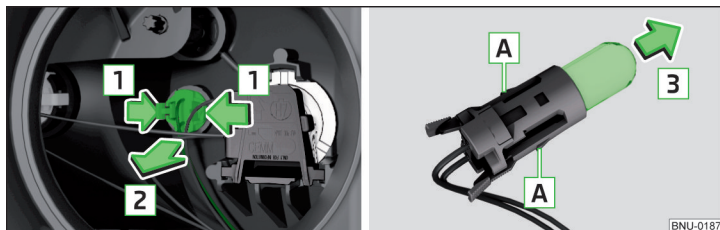
Fig. 339 Înlocuirea becului luminii de poziție
