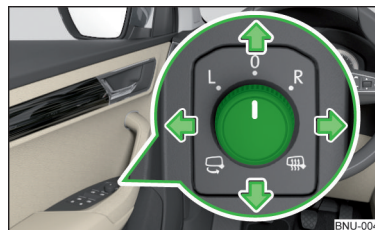
Fig. 73 Operarea oglinzii exterioare
