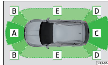
Fig. 253 Zonele baleiate și raza de acțiune a senzorilor
