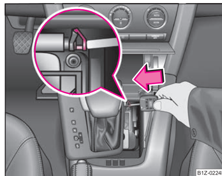
Fig. 140 Deblocarea de urgență a selectorului de viteze
