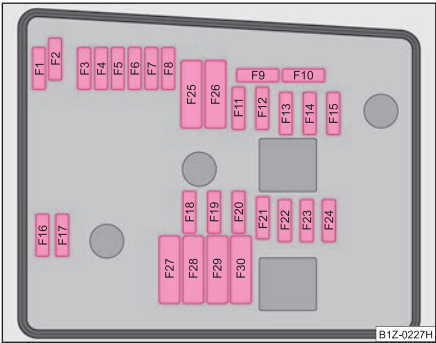
Fig. 220 Prezentare schematică a cutiei cu siguranțe din compartimentul motorului - Varianta 2
