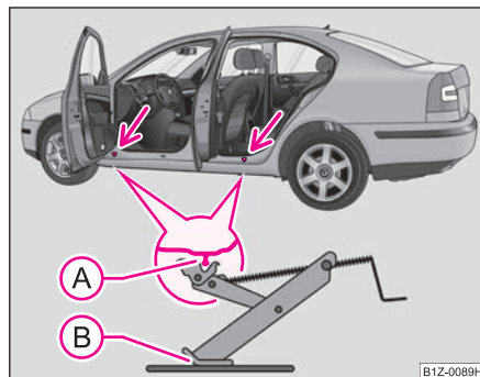
Fig. 210 Înlocuirea roții: Puncte pentru fixarea cricului
