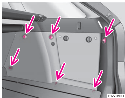
Fig. 72 Portbagajul: Inelele de prindere (Combi)
