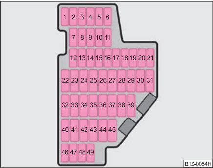
Fig. 221 Prezentare schematică a cutiei cu siguranțe din tabloul de bord
