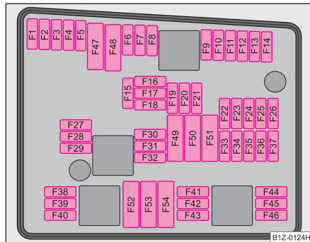
Fig. 219 Prezentare schematică a cutiei cu siguranțe din compartimentul motorului - Varianta 1
