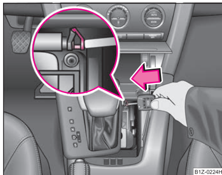
Fig. 145 Deblocarea de urgență a selectorului de viteze
