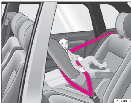
Fig. 174 Scaunul pentru copii corespunzător grupei 0 / 0+
