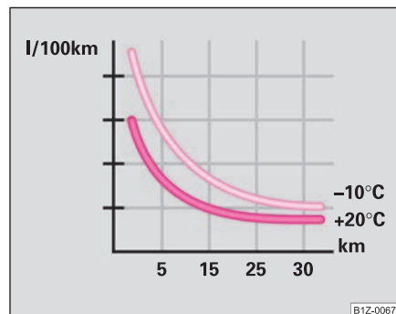
Fig. 185 Consumul de carburant în l/100 km la diverse temperaturi ►
