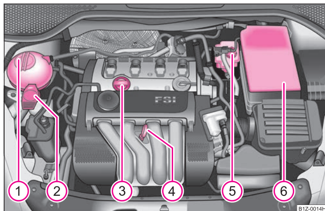
Fig. 192 Motorul pe benzină 1,6 l/85 kW
