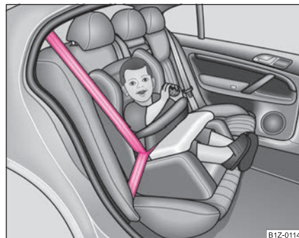
Fig. 175 Scaun cu măsura de siguranță din grupa 1 montat pe bancheta din spate, cu fața la sensul de mers. ►
