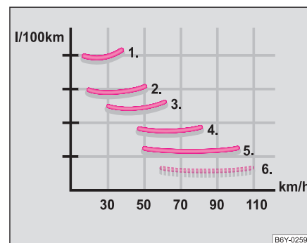
Fig. 183 Consumul de carburant în l/100 km și viteză în km/h
