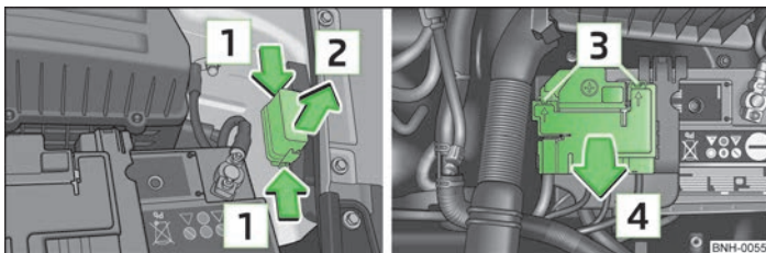
Fig. 125 Bateria autovehiculului: capacul panoului de siguranțe (varianta 2)
