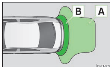
Fig. 67 Asistență la parcare: Raza de acțiune a senzorilor
