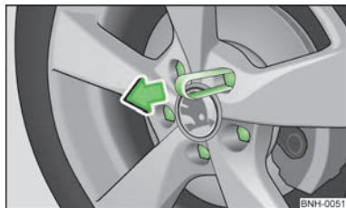
Fig. 108 Scoaterea capacului
