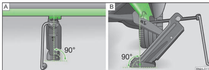
Fig. 114 aplicarea cricului
