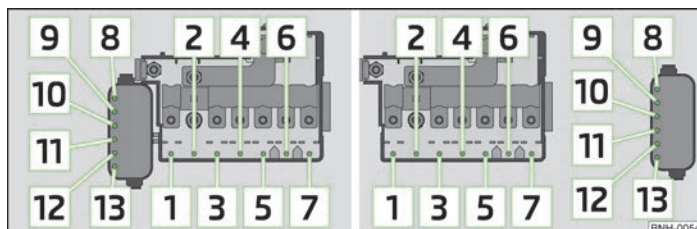
Fig. 123 Reprezentarea schematică a panoului de siguranțe din compartimentul motor: Varianta 1 / varianta 2
