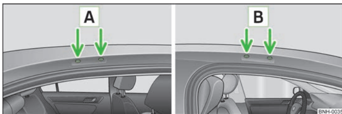
Fig. 42 Puncte de fixare ale suportului principal
