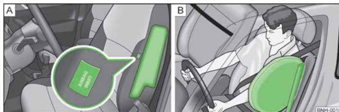
Fig. 84 Locul de amplasare a airbagului lateral în scaunul șoferului/ airbag lateral umplut cu gaz
