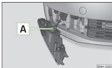
Fig. 131 Înlocuirea becului
