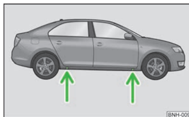
Fig. 113 Înlocuirea roții: Puncte pentru fixarea cricului
