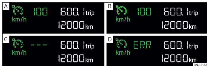
Fig. 121 Afișajul segment: Exemple de afișări de stare a sistemului de menținere automată a vitezei de deplasare (GRA)
