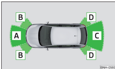
Fig. 116 Zonile supuse sesizării și raza de acțiune a senzorilor
