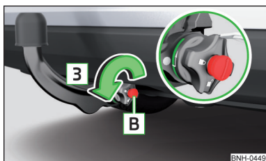
Fig. 137 Descuierea încuietorii
