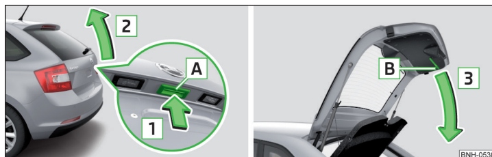
Fig. 40 Deschiderea/inchiderea capotei portbagajului
