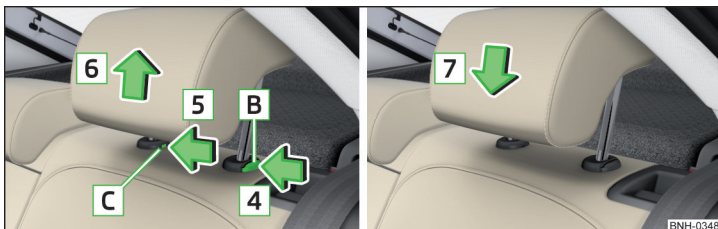
Fig. 60 Tetiere spate: demontarea/montarea
