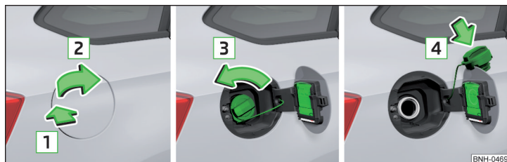
Fig. 142 Deschiderea clapetei rezervorului de combustibil/Deșurubarea bușonului rezervorului de combustibil/Introducerea bușonului rezervorului de combustibil în clapeta rezervorului de combustibil
