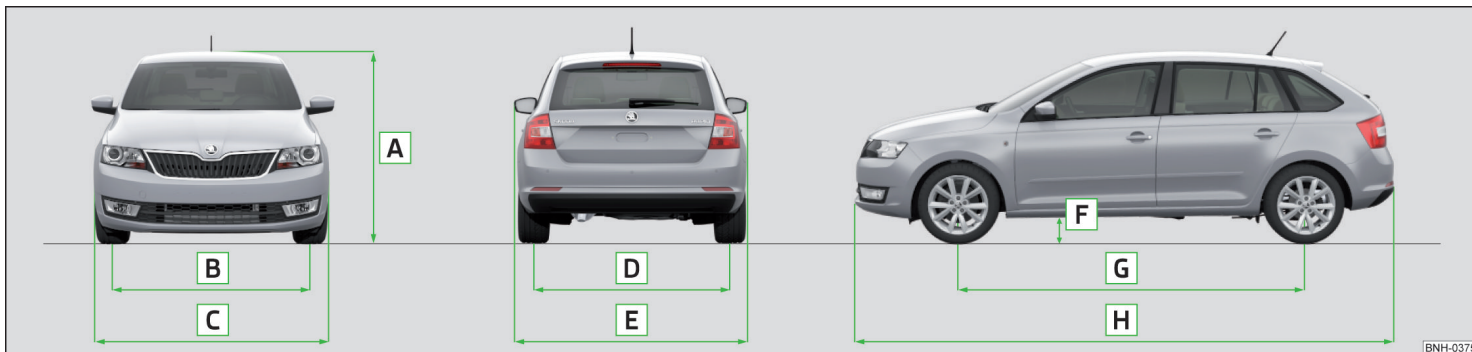
Fig. 190 Prezentarea în principiu: dimensiunile autovehiculului
