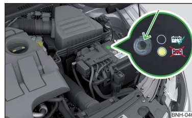
Fig. 150 Bateria autovehiculului: Indicatorul nivelului electrolitului
