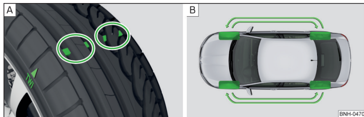
Fig. 152 Prezentarea în principiu: profilul de anvelopă cu urme de uzură / permutarea roților
