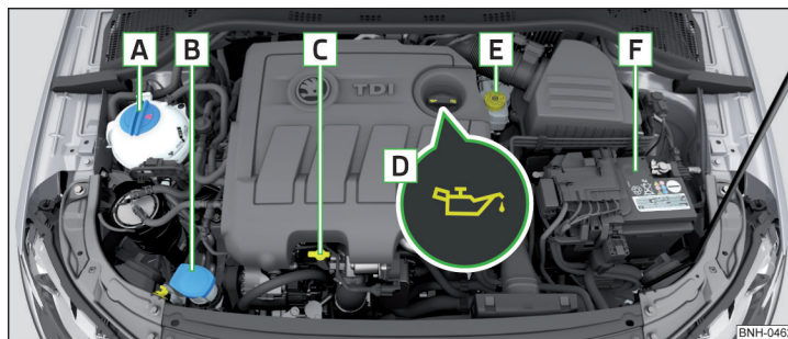
Fig. 144 Prezentarea în principiu: Compartimentul motor
