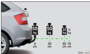
Fig. 139 Prezentarea proeminenței maxime admise a cuplei sferice de pe dispozitivul de tractare și a masei totale admise a accesoriilor, incl. a sarcinii în funcție de poziția centrului de greutate a încărcăturii.
