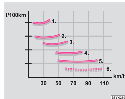
Fig. 148 Consumul de carburant în l/100 km și viteză în km/h
