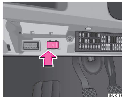
Fig. 33 Compartimentul siguranțelor: Înterupătorul pentru lumina de zi
