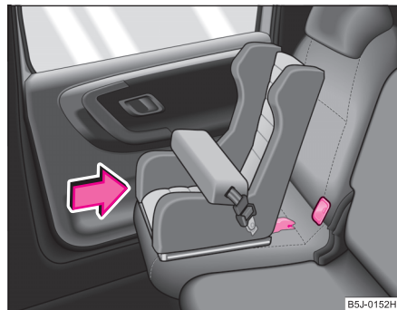
Fig. 143 Scaunul cu sistem ISOFIX se montează în dispozitivele de prindere existente.
