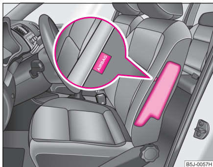
Fig. 129 Scaunul conducătorului: Amplasarea airbag-urilor
