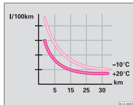
Fig. 150 Consumul de carburant în l/100 km la diverse temperaturi
