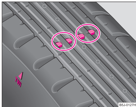
Fig. 164 Profilul pneului cu indicator de uzură
