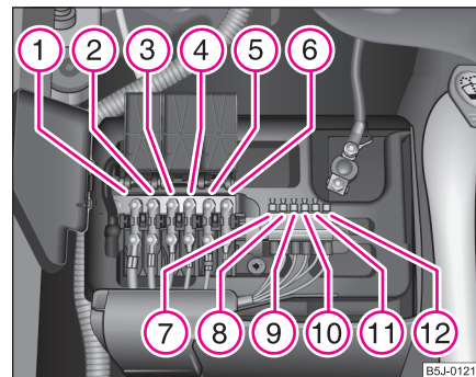
Fig. 182 Reprezentare schematică a dispunerii siguranțelor de pe baterie
