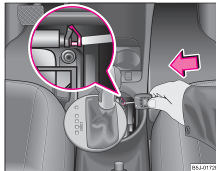
Fig. 109 Deblocarea de urgență a selectorului de viteze
