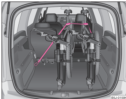
Fig. 71 Asigurarea bicicletei cu o centură
