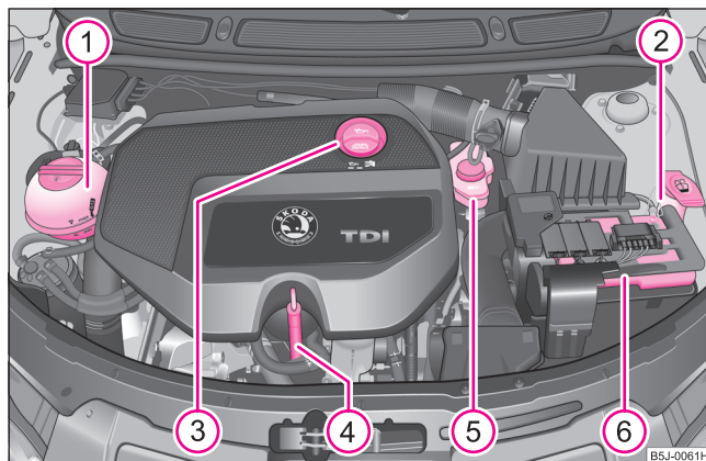
Fig. 156 Motorul diesel 1,9 l/77 kW
