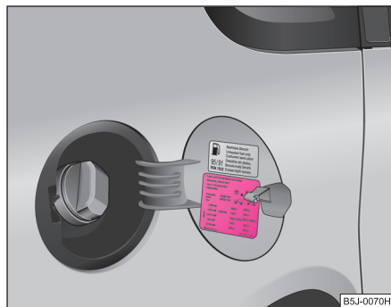
Fig. 163 Clapeta rezervorului deschisă și tabelul cu datele referitoare la presiune
