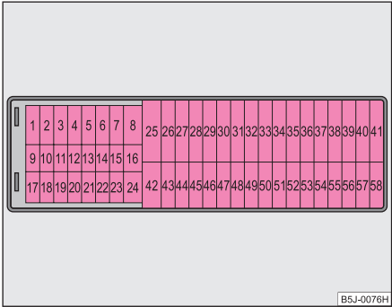
Fig. 179 Prezentare schematică a suporțului de siguranțe
