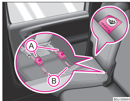
Fig. 142 Inelele de prindere (sistemul ISOFIX)
