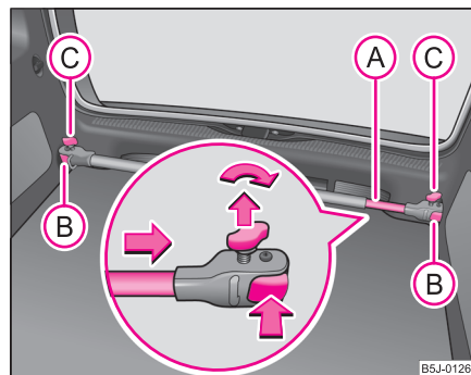
Fig. 66 Montarea suportului transversal
