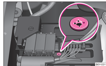
Fig. 162 Bateria cu indicator al nivelului de încărcare
