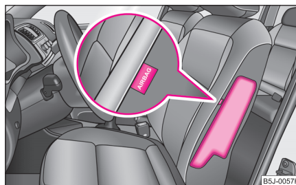
Fig. 129 Scaunul conducătorului: Amplasarea airbag-urilor
