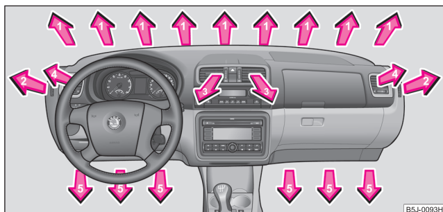
Fig. 94 Gurile de ventilație a aerului
