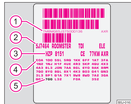
Fig. 203 Plăcuța cu datele autovehiculului
