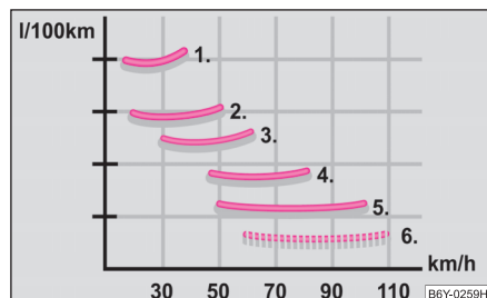
Fig. 149 Consumul de carburant în l/100 km și viteza în km/h
