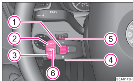
Fig. 110 Modul multifuncțional: Taste pentru comanda radio
