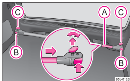
Fig. 65 Montarea suportului transversal
