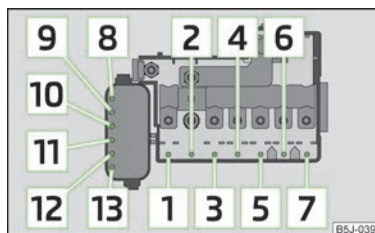
Fig. 141 Bateria autovehiculului: Capacul panoului de siguranțe
