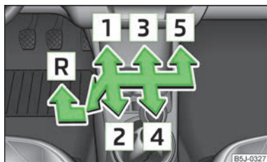
Fig. 82 Schema de selectare a treptelor cutiei de viteze manuale cu 5 trepte
