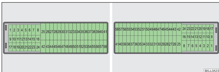
Fig. 140 Reprezentare schematică a panoului de siguranțe pentru autovehiculele cu volanul pe stânga / dreapta
