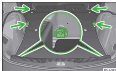
Fig. 154 Portbagajul: Inele de prindere
