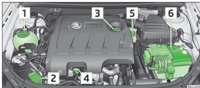
Fig. 115 Motorul diesel 1.6l/77 kW
