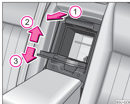
Fig. 78 Montarea cutiei frigorifice
