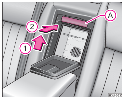
Fig. 77 Demontarea cutiei frigorifice
