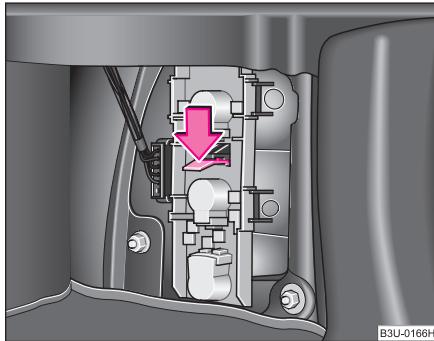
Fig. 199 Portbagajul: Demontarea suportului becurilor cu incandescență
