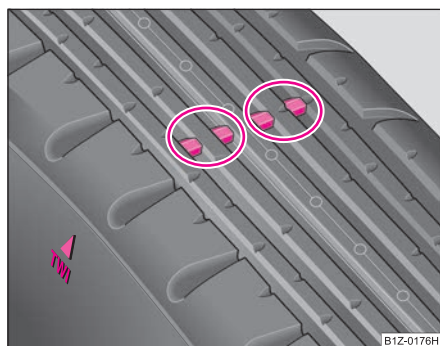
Fig. 181 Profilul pneului cu indicator de uzură
