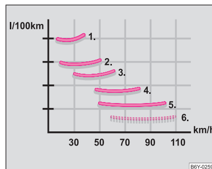
Fig. 162 Consumul de carburant în l/100 km și viteza în km/h
