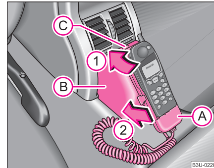
Fig. 131 Adaptare universală pentru telefon spate
