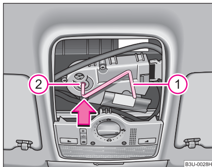
Fig. 34 Plafonul: Acționarea în caz de urgență
