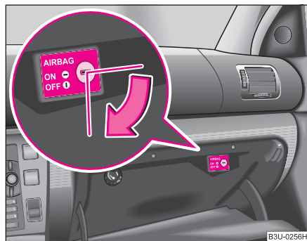
Fig. 149 Torpedoul: Comutatorul pentru airbag-urile pasagerului dreapta
