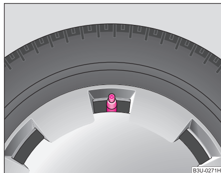
Fig. 180 Roată cu capac de roată și supapă prelungită.
