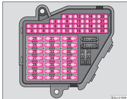
Fig. 198 Prezentare schematică a suportului de siguranțe
