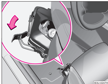
Fig. 185 Scaun față: Extinctorul de incendii
