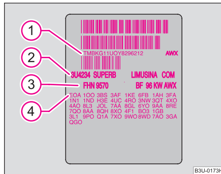
Fig. 207 Plăcuța cu datele autovehiculului
