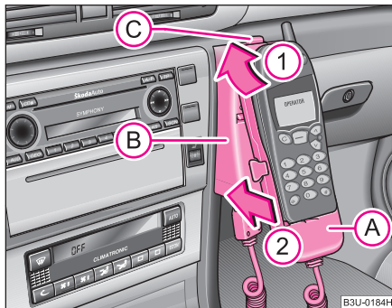
Fig. 130 Adaptare universală pentru telefon față
