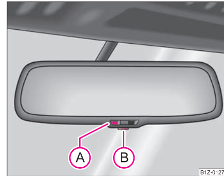
Fig. 52 Oglinda interioară cu reglare automată antiiorbire
