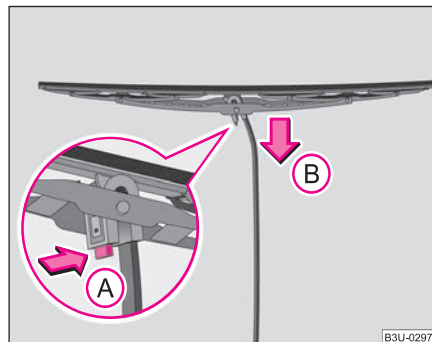
Fig. 51 Lamela ștergătorului de parbriz
