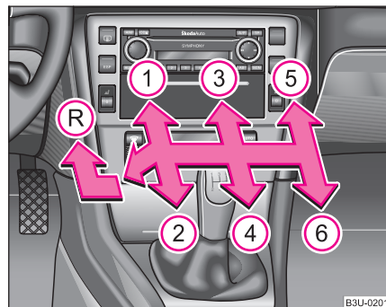
Fig. 117 Schemă de comutare la autovehiculele cu transmisie manuală cu 6 viteze
