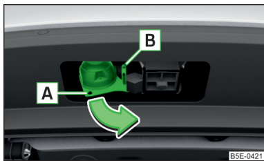
Илл. 197 Откидывание 13-контактной розетки, стопорная проушина
