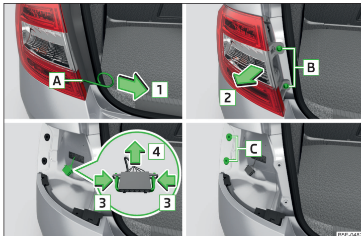
Илл. 250 Снятие фонаря / отсоединение разъёма
