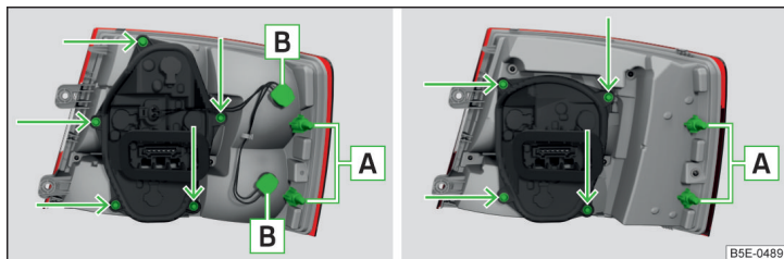
Илл. 251 Наружная часть заднего фонаря: фонарь с лампами / фонарь со светодиодами
