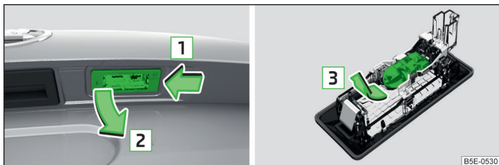
Илл. 249 Снятие плафона освещения номерного знака / замена лампы накаливания
