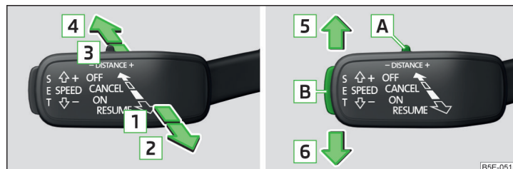
Илл. 171 Рычаг управления
