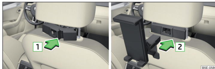
Илл. 105 Размещение адаптера / установка держателя
