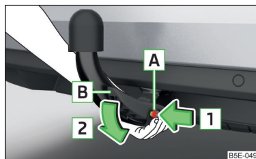
Илл. 195 Снятие шарового наконечника
