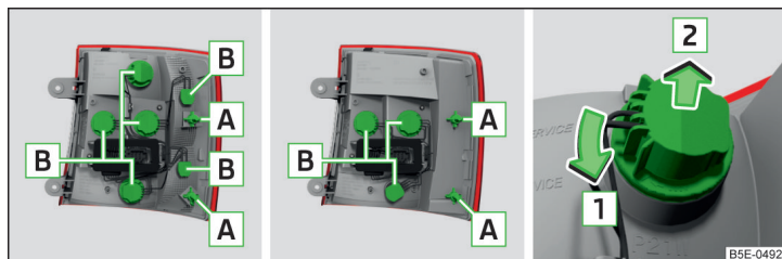
Илл. 253 Наружная часть заднего фонаря: фонарь с лампами / фонарь со светодиодами
