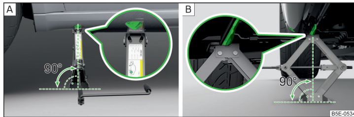
Илл. 222 Условное изображение: установка домкрата
