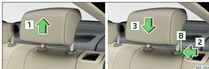
Илл. 74 Задний подголовник: перемещение вверх/вниз
