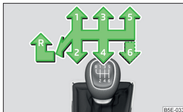
Илл. 148 Схема переключения передач 5-ступенчатой и 6-ступенчатой механических коробок передач
