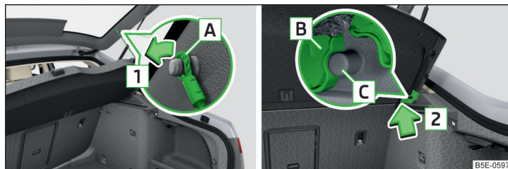
Илл. 118 Снятие полки багажного отсека
