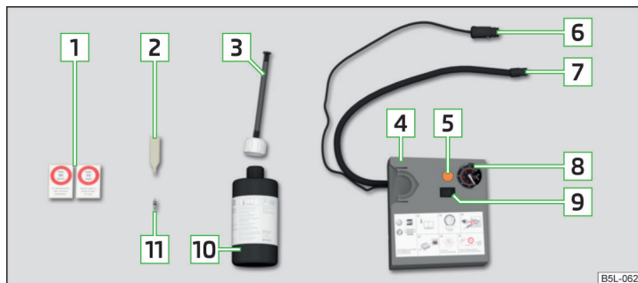
Илл. 223 Условное изображение: состав комплекта для ремонта шин
