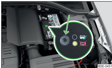
Илл. 210 Аккумуляторная батарея: индикатор уровня электролита
