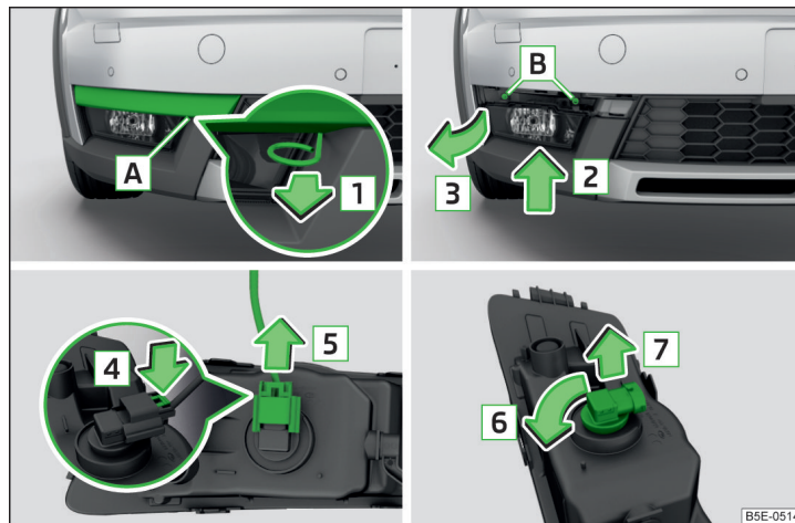
Илл. 248 Снятие противотуманной фары / замена лампы накаливания: вариант 2
