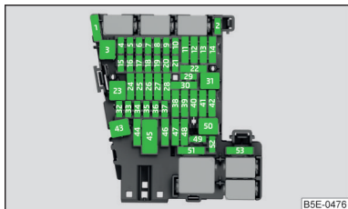
Илл. 240 Предохранители
