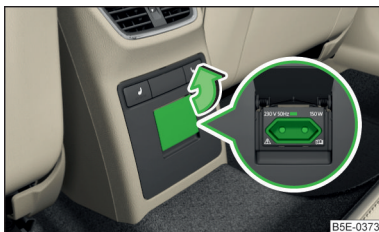
Илл. 102 Открытие крышки розетки на 230 В
