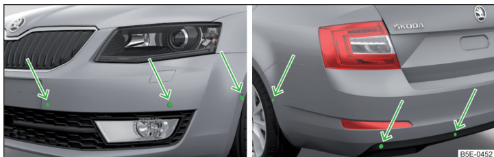
Илл. 157 Место установки датчиков с левой стороны автомобиля: спереди/сзади
