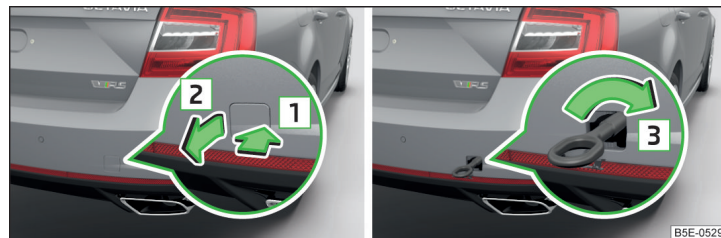
Илл. 229 Снятие крышки / установка буксирной проушины: вариант 2
