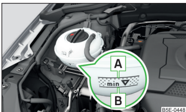
Илл. 207 Расширительный бачок ОЖ
