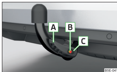
Илл. 192 Правильно закреплённый шаровой наконечник
