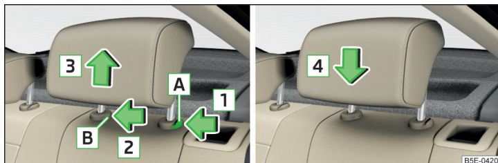
Илл. 75 Задний подголовник: снятие/установка
