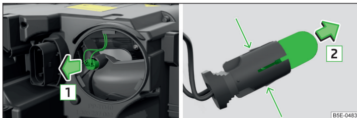
Илл. 246 Ксеноновая фара: лампа накаливания для дополнительного габаритного фонаря
