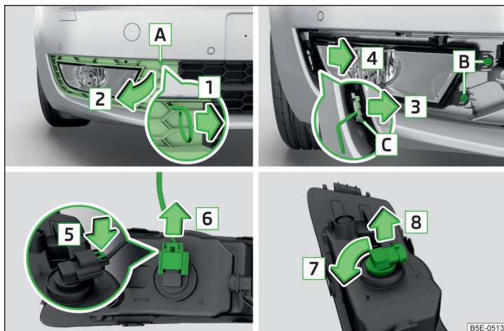
Илл. 247 Снятие противотуманной фары / замена лампы накаливания: вариант 1
