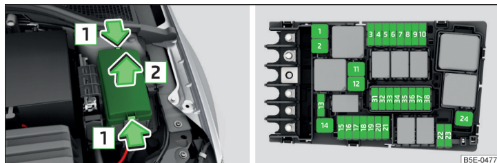
Илл. 241 Снятие крышки блока предохранителей / предохранители
