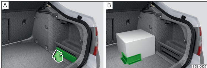
Илл. 123 Извлечение элемента Cargo / пример фиксации груза с помощью элемента Cargo
