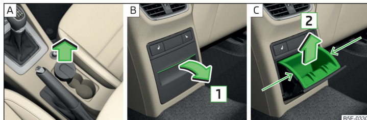
Илл. 91 Снятие передней пепельницы / открытие задней пепельницы / снятие вставки задней пепельницы
