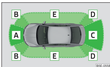
Илл. 158 Зона чувствительности и дальность действия датчиков
