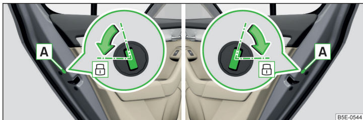
Илл. 233 Аварийное запираение задняя левая/правая дверь
