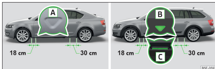
Илл. 221 Опорные точки под домкрат: вариант 1 / вариант 2
