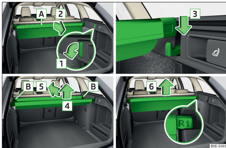
Илл. 125 Многофункциональный карман: выдвигание / установка / складывание / снятие
