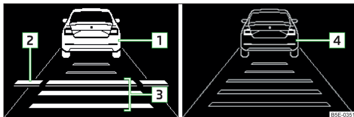
Илл. 169 Дисплей в комбинации приборов: пример для индикации адаптивного круиз-контроля
