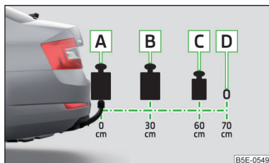
Илл. 196 Максимально допустимый вылет шарового наконечника ТСУ с указанием разрешённой полной массы установленного аксессуара и его груза в зависимости от расположения центра тяжести груза
