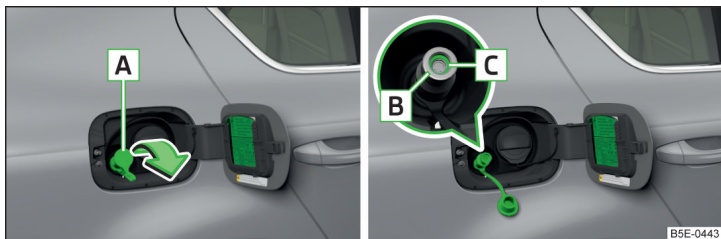
Илл. 201 Заправочный штуцер
