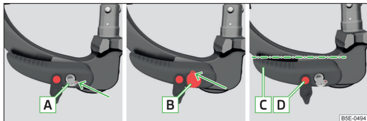
Илл. 188 Положение готовности к установке: ключ, вариант 1 / ключ, вариант 2 / положение рычага и расцепляющего пальца для обоих вариантов ключа
