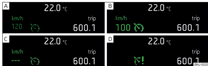
Илл. 166 Дисплей MAXI DOT (монохроматический): пример отображения состояния круиз-контроля
