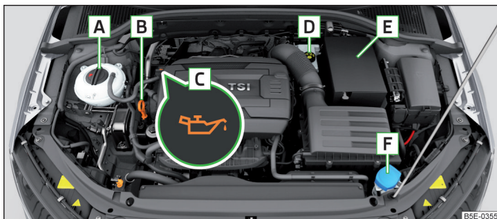
Илл. 204 Условное изображение: моторный отсек
