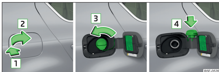
Илл. 199 Открыть лючок / отвернуть пробку заливной горловины / насадить пробку на крышку лючка
