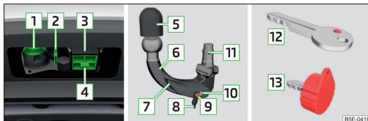
Илл. 185 Поперечина ТСУ / шаровой наконечник / ключ (варианты 1 и 2)
