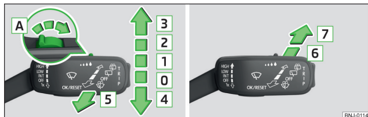
Илл. 68 Переключатель стеклоочистителей и стеклоомывателей: передний/задний
