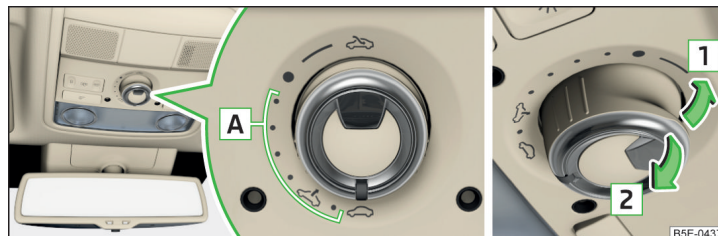
Илл. 50 Управление подъёмно-сдвижным люком: вариант 1
