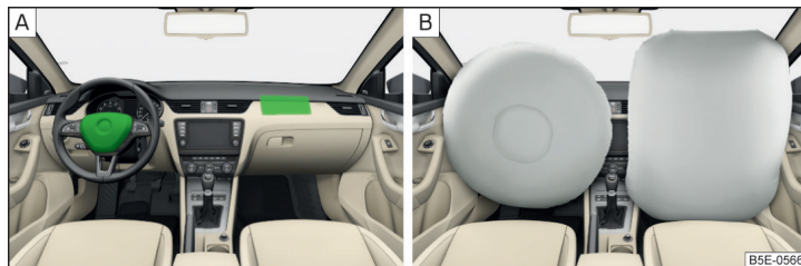
Илл. 8 Места установки подушек безопасности / полностью раскрывшиеся подушки безопасности
