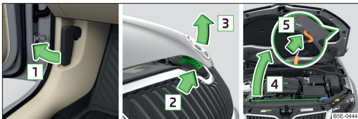
Илл. 203 Открытие капота
