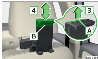
Илл. 108 Подгонка размера захвата
