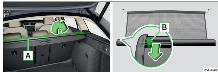
Илл. 130 Раскладывание части сматываемой шторки багажного отсека / рычаг разблокировки
