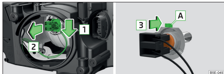
Илл. 244 Галогеновые фары: лампа накаливания ближнего света
